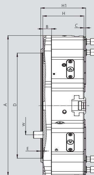
Vorderansicht Id.Nr. 163306
