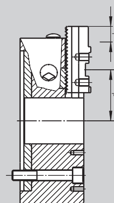
Grundbacke Stellung »p«
