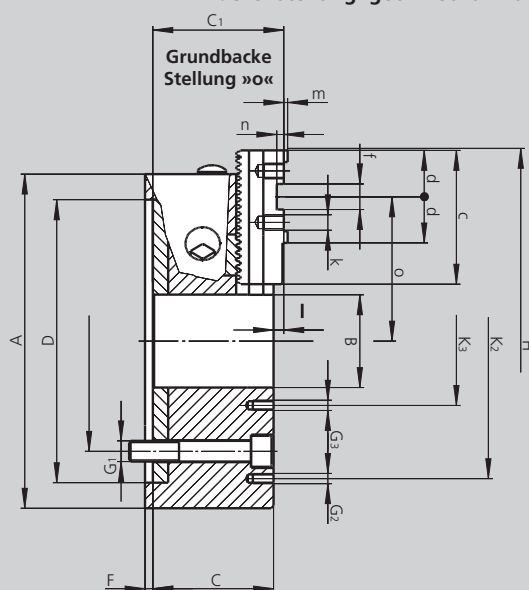
Backenstellung: geöffnet für Außenspannung
