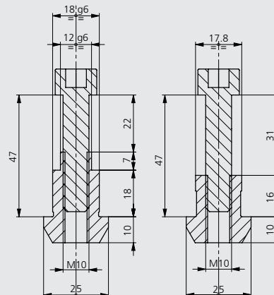
T-SLOT 18 46204102
