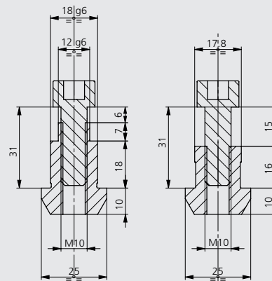
T-SLOT 18 46204105
