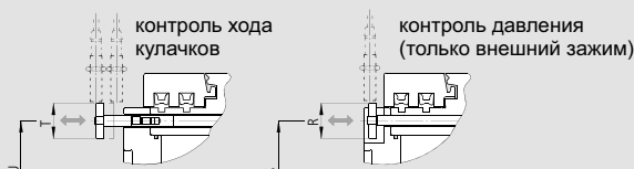
увеличенный чертеж
