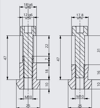
T-SLOT 18 46204102
