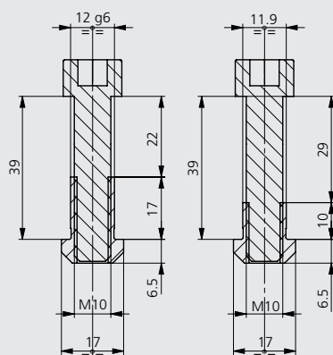
T-SLOT 12 46204100
