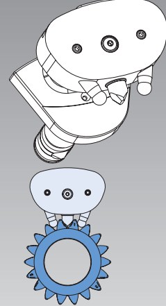
Zahnflankenspannung
