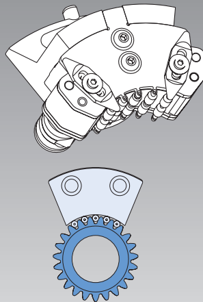
Zahnflankenspannung Rollenkäfig
