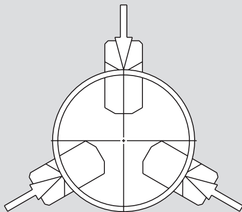
3-Punktspeisung
